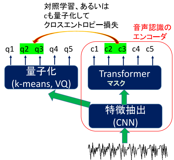
図-3 wav2vec 2.0 / HuBERT の枠組み
