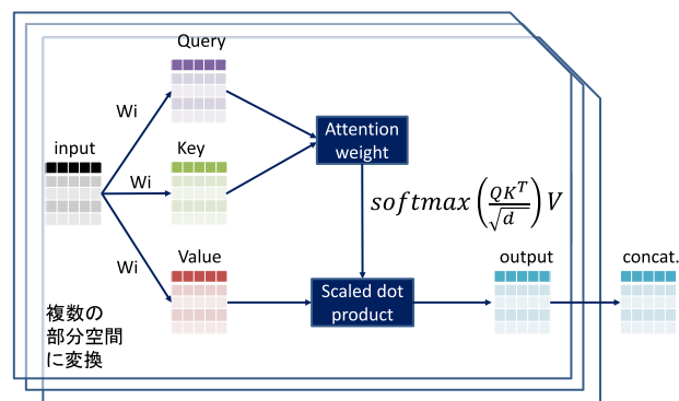
図-1 自己注意機構
