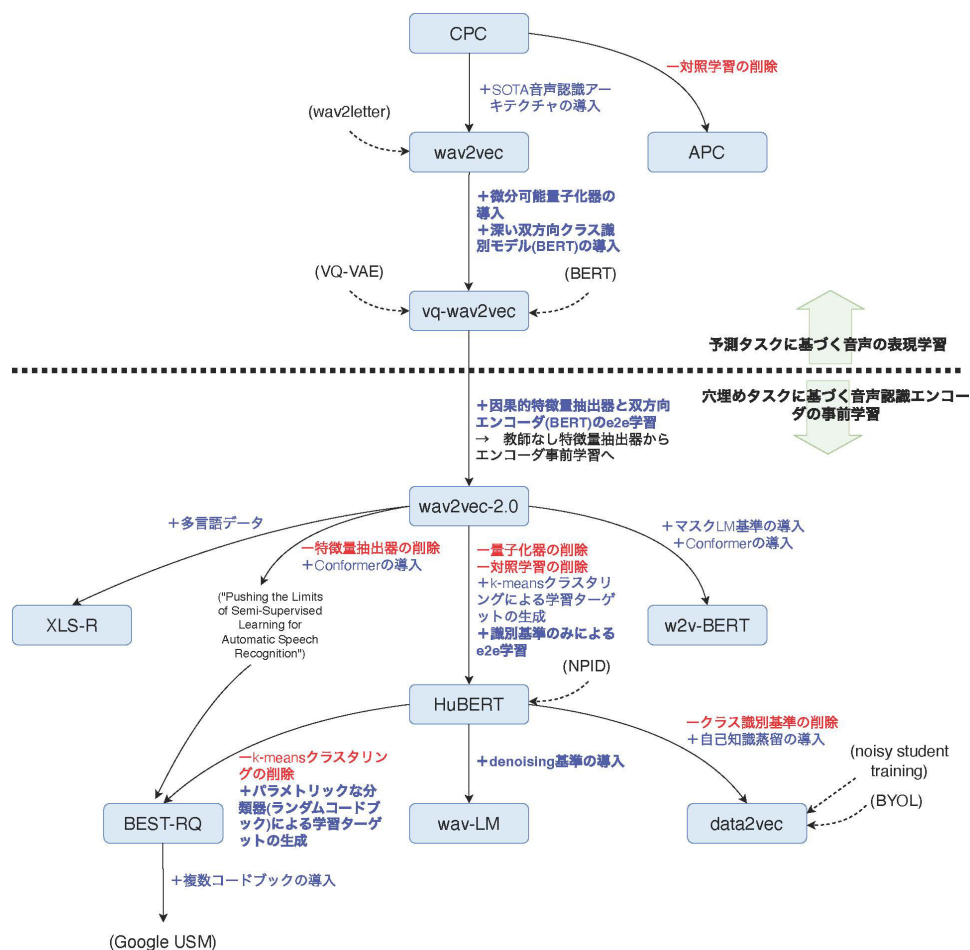
図-4 大規模事前学習モデルの展開
